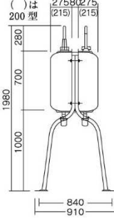
■W型用200・250共通普通脚使用「アイボリー」
