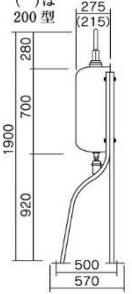
■200・250共通脚「アイボリー」
