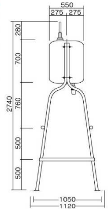
■長脚「アイボリーブラック」
