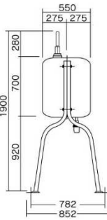
■コンパクト脚「アイボリー」
