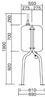
■幅狭脚「ブラック」
